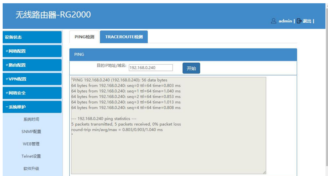
图 4-52 PING 检测
