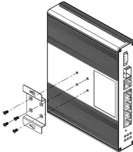
图 2-5 壁挂附件安装示意图
