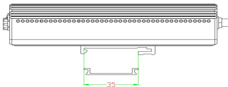
图 2-8 导轨附件尺寸图
