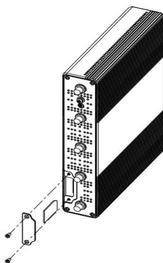
图 2-4 SIM 卡安装示意图
