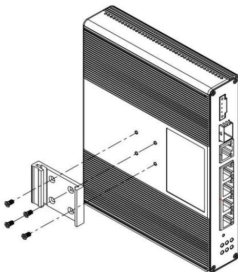
图 2-7 导轨附件安装示意图
